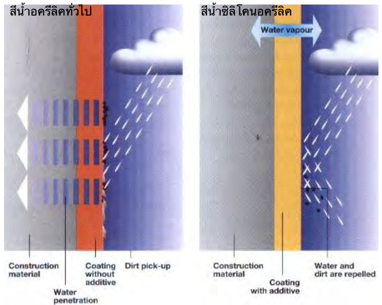
รูปที่ 5: อัตราการซึมของน้ำลงพื้นผิว
